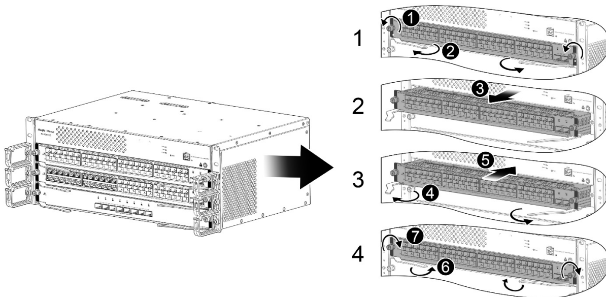
图 7-2 更换业务模块示意图
