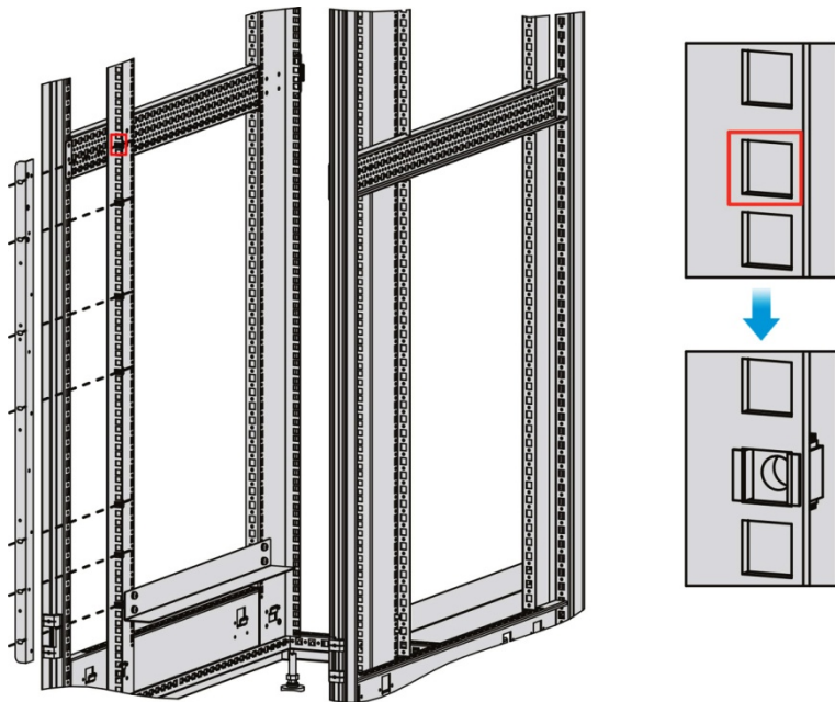
图 3-3 丈量挂耳高度和安装孔示意图
