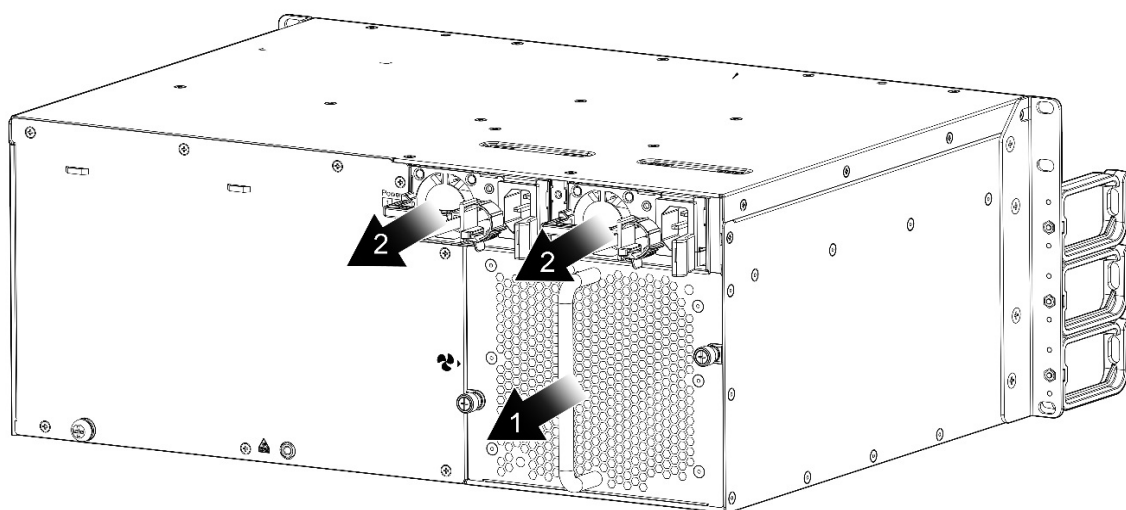
图 1-5 RG-NBS7003 通风散热出风方案图
