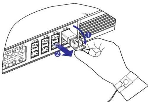
图 7-1 SFP/SFP+光模块拔出示意图
