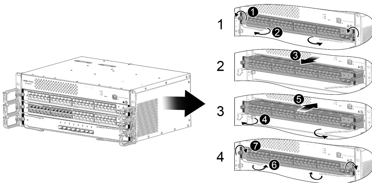
图 3-9 RG-NBS7003 模块安装示意图
