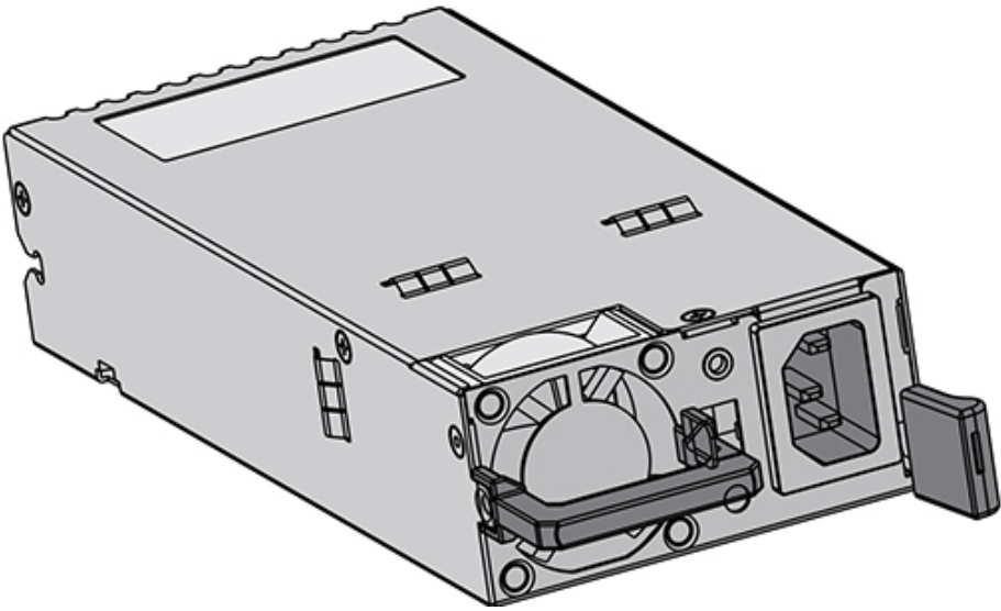
图 1-13 RG-PA460I-FS 模块外观
