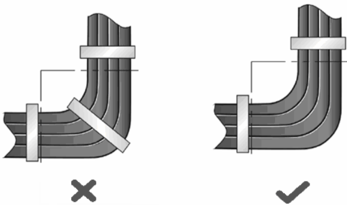
图 D-3 电缆捆扎示意图（三）
