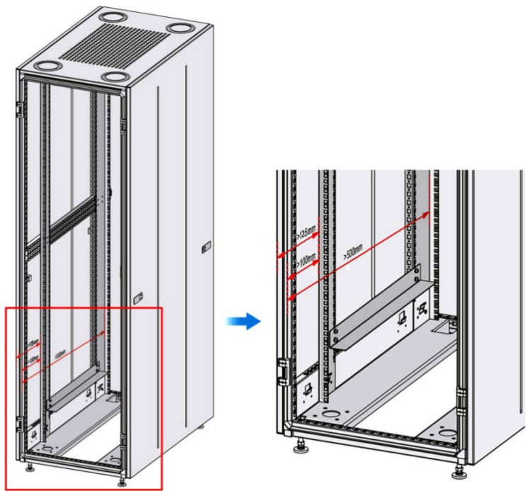
图 2-3 机柜尺寸要求示意图
