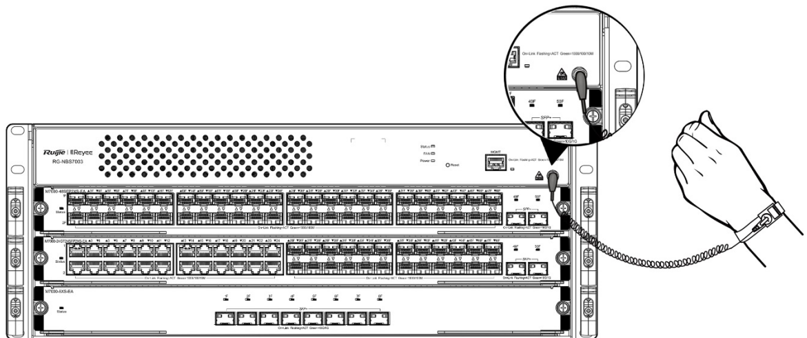
图 2-1 RG-NBS7003 防静电方式示意图
