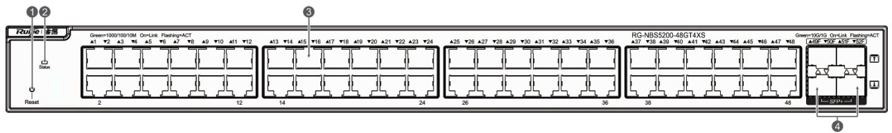
图 1-10 RG-NBS5200-48GT4XS 前面板示意图
