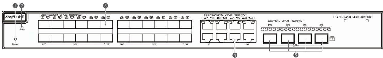
图 1-6 RG-NBS5200-24SFP/8GT4XS 前面板示意图
