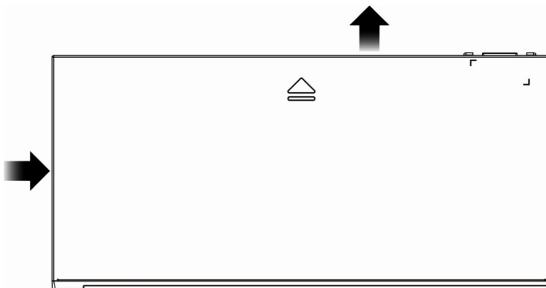
图 1-4 RG-NBS5200-24GT4XS 通风散热对流方案
