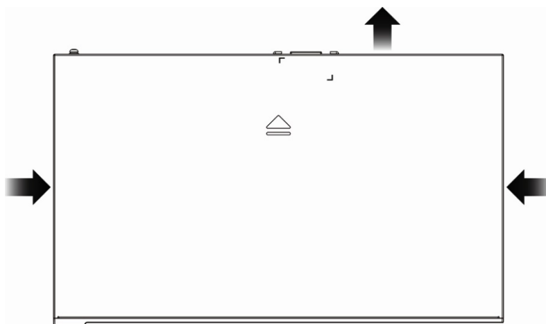
图 1-12 RG-NBS5200-48GT4XS 通风散热对流方案
