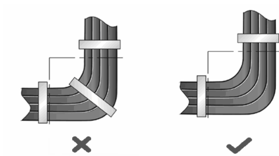
图 D-3 电缆捆扎示意图（三）
