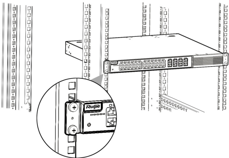
图 3-3 机柜式挂耳安装示意图三
