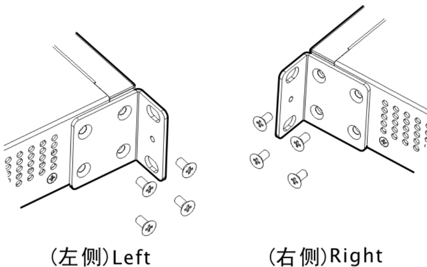
图 3-1 机柜式挂耳安装示意图一
