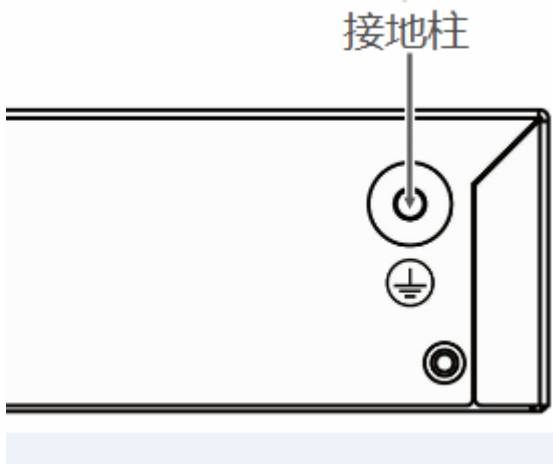
图2-1 RG-NBS5200 系列交换机接地示意图
