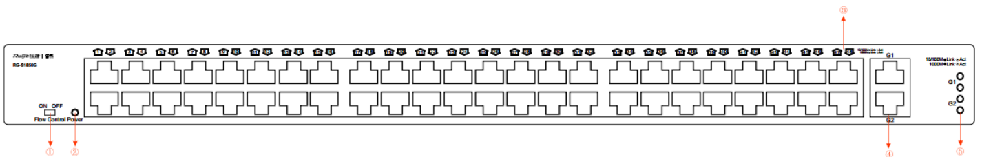
图 1-2 RG-S1850G 前面板示意图
