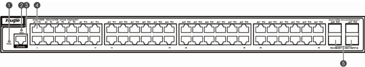
图 1-5 RG-NBS5710-48GT4SFP-E 前面板示意图
