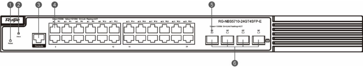
图 1-2 RG-NBS5710-24GT4SFP-E 前面板示意图
