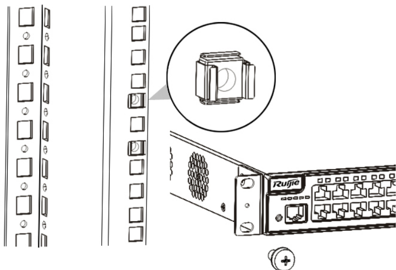
图 3-3 机柜式挂耳安装示意图三
