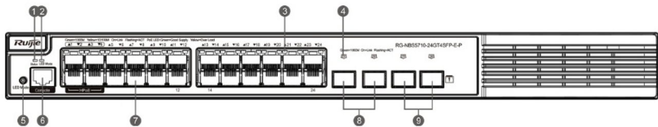
图 1-9 RG-NBS5710-24GT4SFP-E-P 前面板示意图
