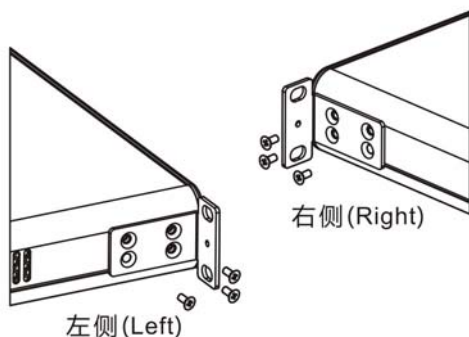
图 3-2 24 口设备机柜式挂耳安装示意图一
