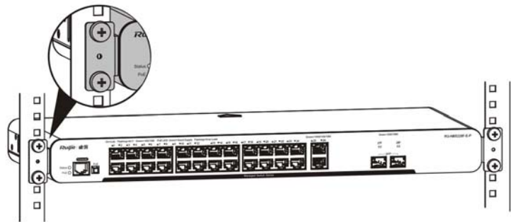
图 3-6 24 口设备机柜式挂耳安装示意图三
