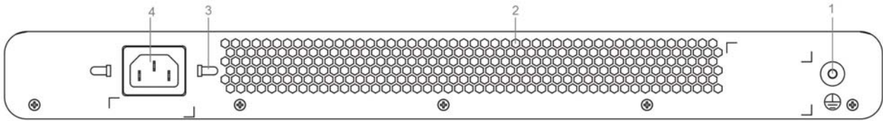
图 1-21 RG-NBS228F-E、RG-NBS228F-S 后面板图
