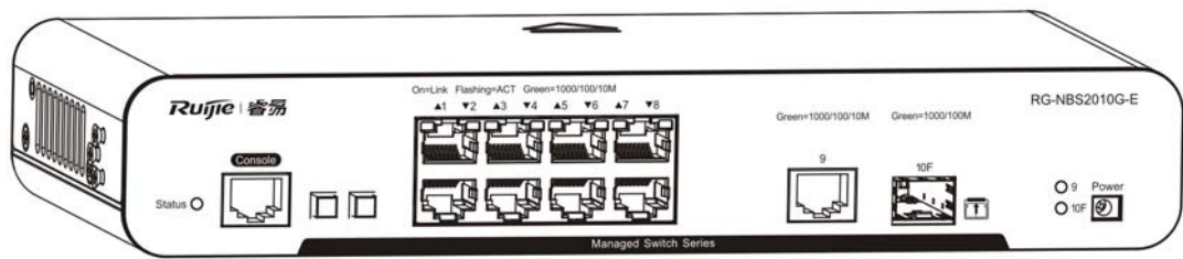
图 1-9 RG-NBS2010G-E 产品外观图
