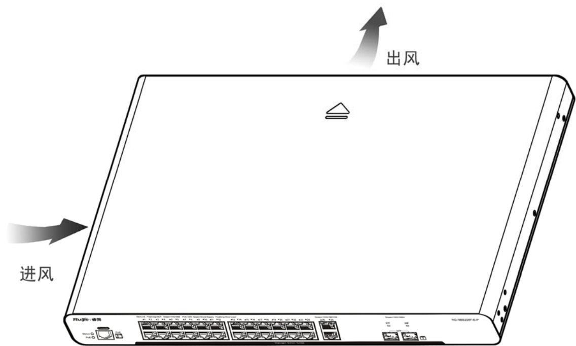
图 1-38 RG-NBS2028G-E-LP 通风散热对流方案图
