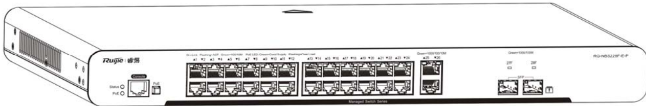
图 1-26 RG-NBS228F-E-P 产品外观图
