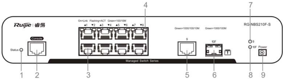
图 1-4 RG-NBS210F-S 前面板图
