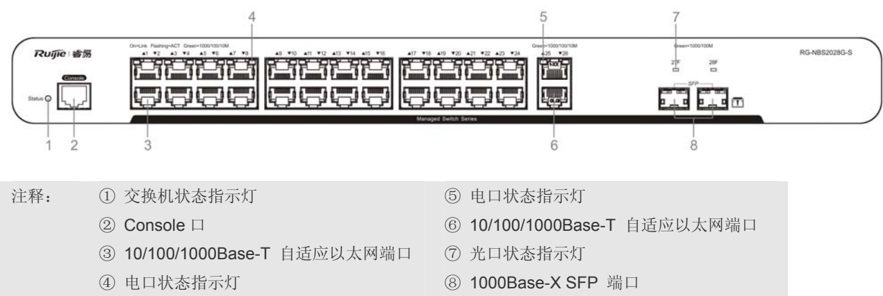
图 1-33 RG-NBS2028G-S 前面板图
