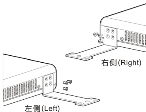
图 3-8 24 口设备挂壁式挂耳安装示意图一
