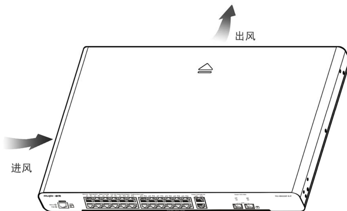
图 1-42 RG-NBS2028G-E-P 通风散热对流方案图
