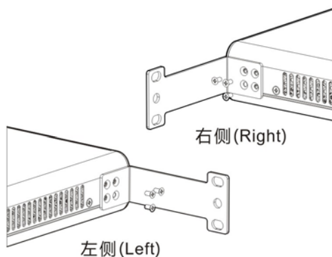
图 3-1 8 口设备机柜式挂耳安装示意图一
