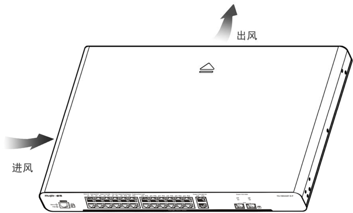
图 1-29 RG-NBS228F-E-P 通风散热对流方案图
