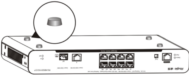
图 3-11 桌面式安装示意图一
