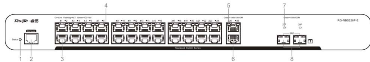
图 1-19 RG-NBS228F-E 前面板图
