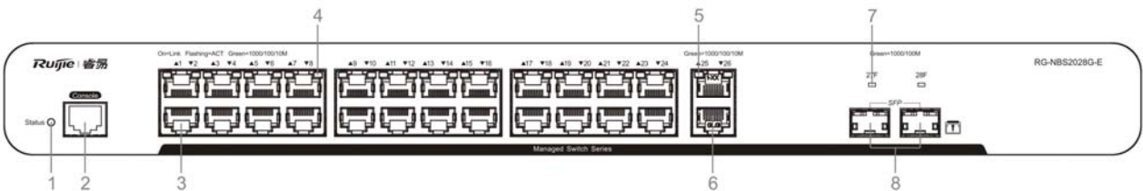
图 1-32 RG-NBS2028G-E 前面板图
