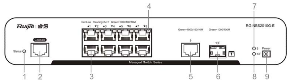
图 1-11 RG-NBS2010G-E 前面板图
