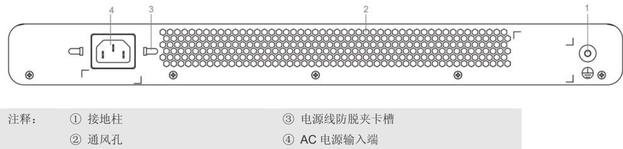
图 1-34 RG-NBS2028G-E、RG-NBS2028G-S 后面板图
