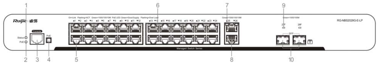
图 1-36 RG-NBS2028G-E-LP 前面板图
