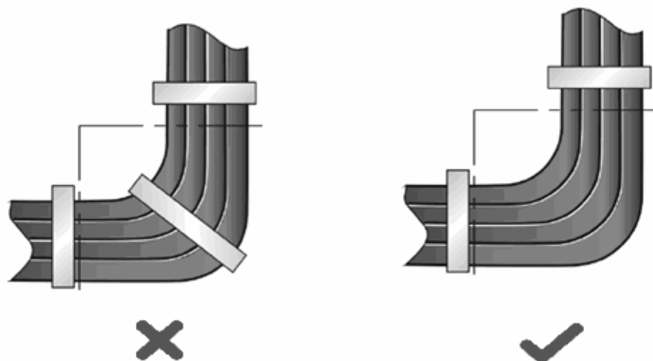
图 D-3 电缆捆扎示意图（三）
