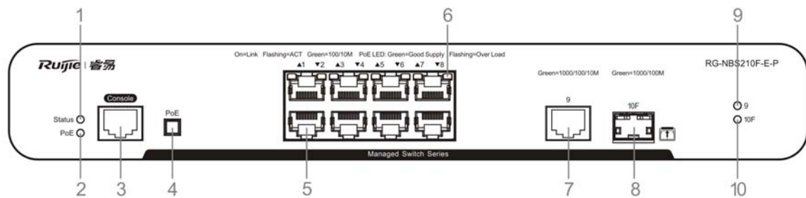
图 1-7 RG-NBS210F-E-P 前面板图
