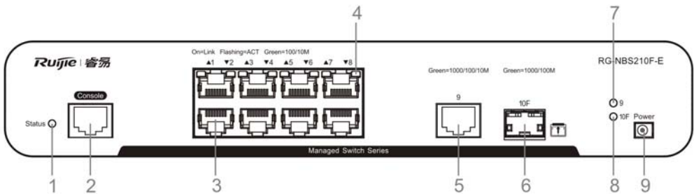
图 1-3 RG-NBS210F-E 前面板图
