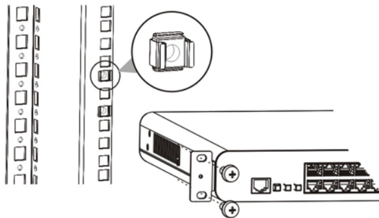
图 3-5 8 口设备机柜式挂耳安装示意图三
