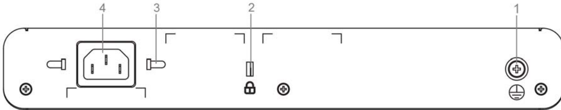
图 1-16 RG-NBS2010G-E-P 后面板图
