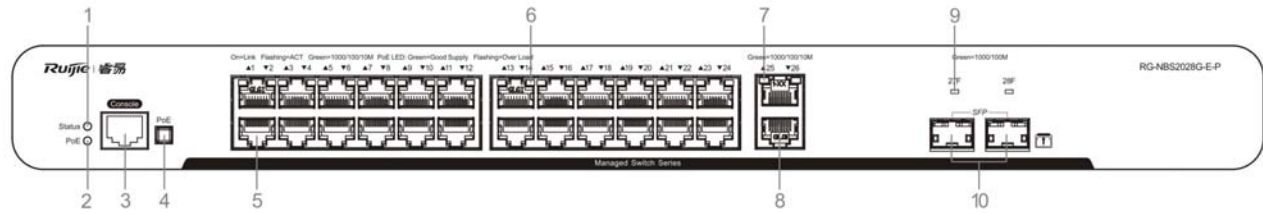
图 1-40 RG-NBS2028G-E-P 前面板图
