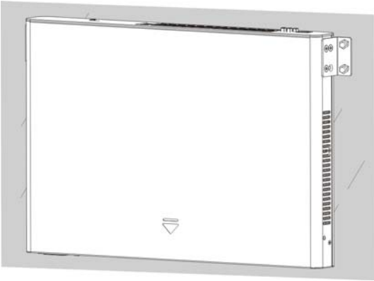
图 3-10 24 口设备挂壁式挂耳安装示意图二
