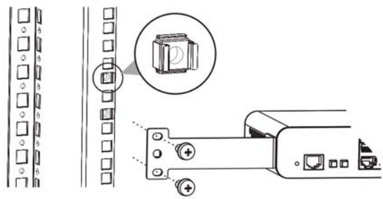
图 3-4 24 口设备机柜式挂耳安装示意图二
