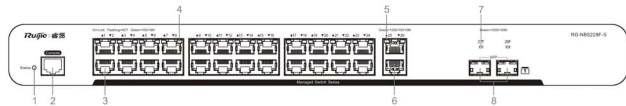
图 1-20 RG-NBS228F-S 前面板图
