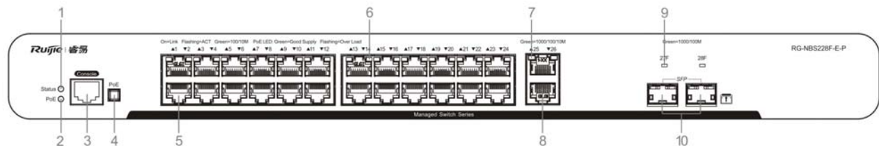
图 1-27 RG-NBS228F-E-P 前面板图
