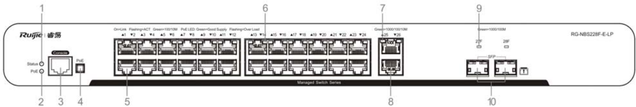
图 1-23 RG-NBS228F-E-LP 前面板图
