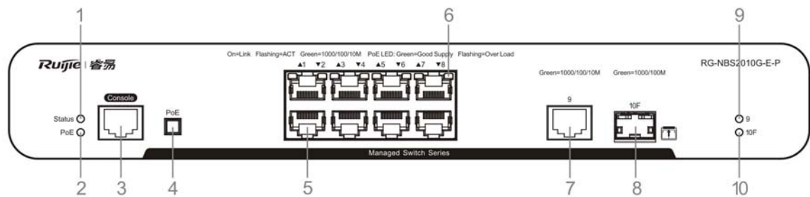
图 1-15 RG-NBS2010G-E-P 前面板图
