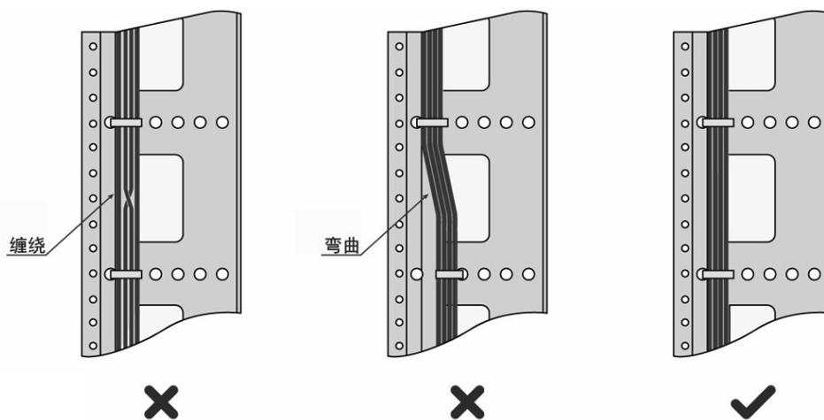
图 B-1 电缆捆扎示意图（一）
