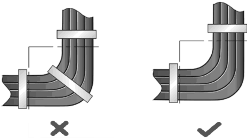
图 B-3 电缆捆扎示意图（三）
