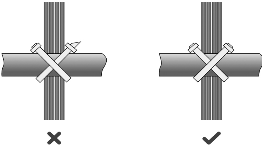
图 B-2 电缆捆扎示意图（二）
