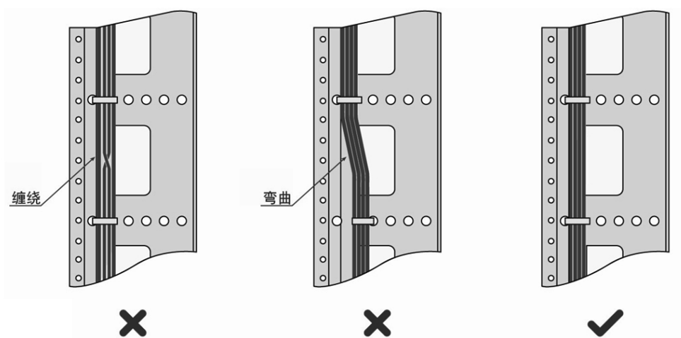
图 B-1 电缆捆扎示意图（一）
