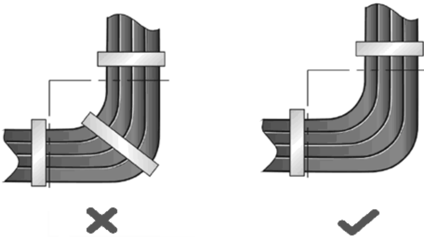
图 B-3 电缆捆扎示意图（三）
