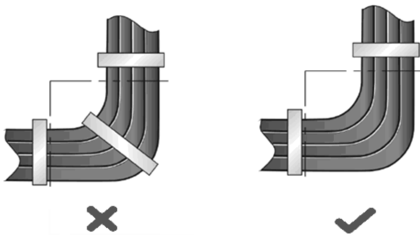
图 B-3 电缆捆扎示意图（三）
