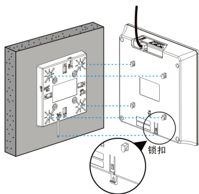
图 3-8 将 AP 扣入挂架
