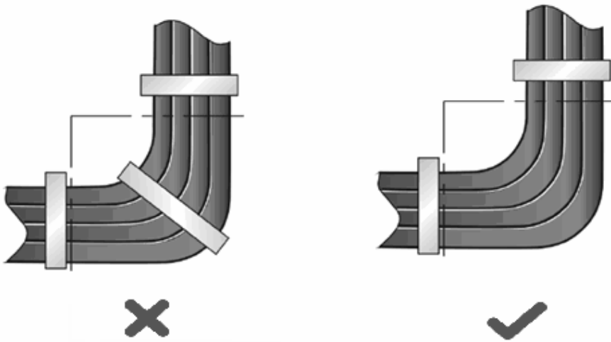
图 D-3 电缆捆扎示意图（三）
