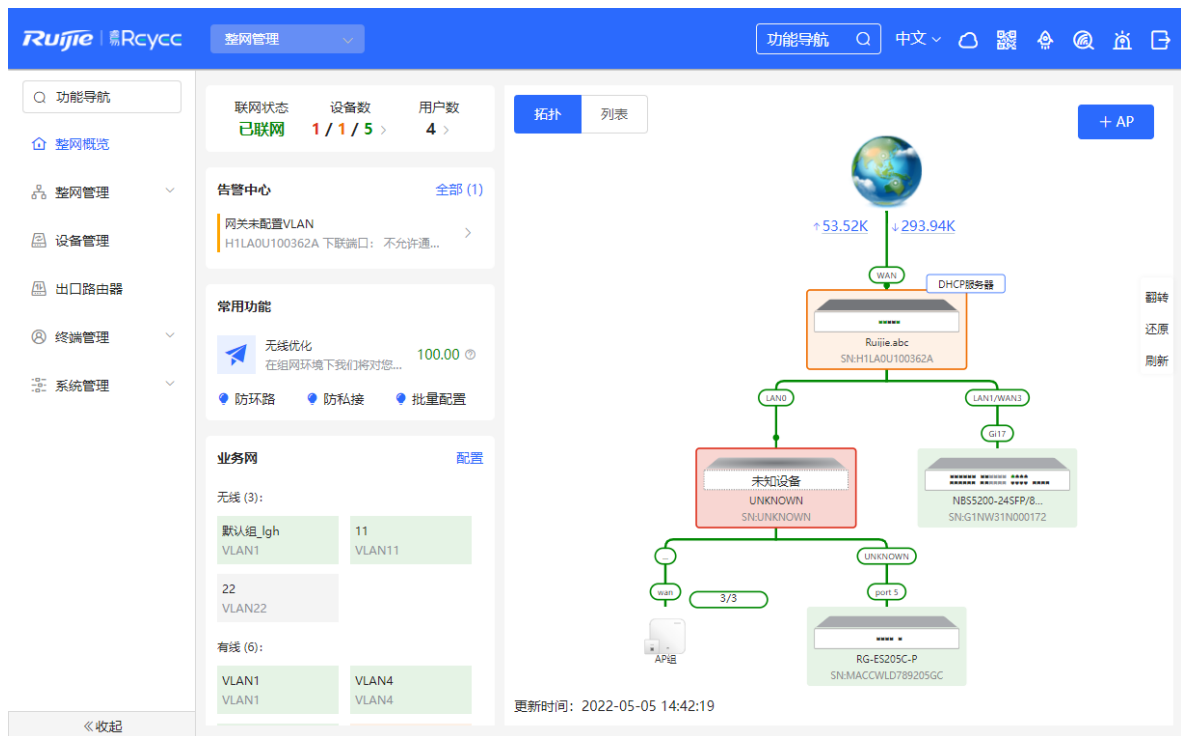
图1-2 组网模式下整网管理模式 Web 页面
