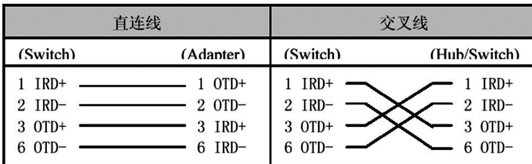
图 A-3100BASE-TX/10BASE-T 双绞线联接方式
