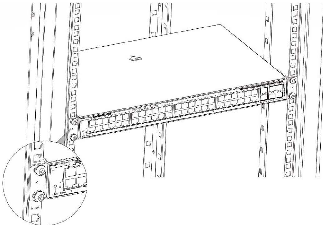
图3-3 机柜式挂耳安装示意图三
