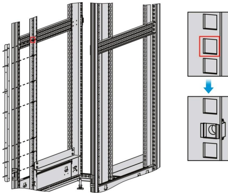
图3-2 机柜式挂耳安装示意图二
