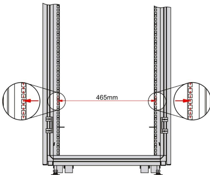
图2-1 19英寸标准机柜示意图
