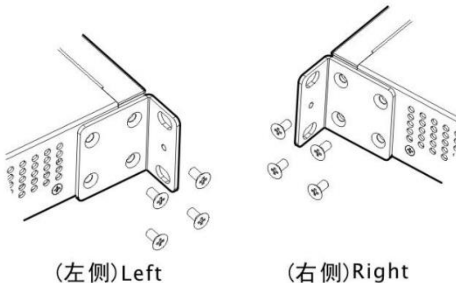
图3-1 机柜式挂耳安装示意图一
